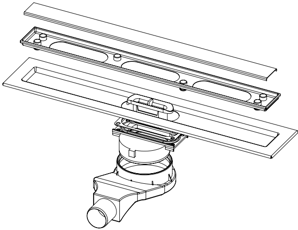
Perspektif
