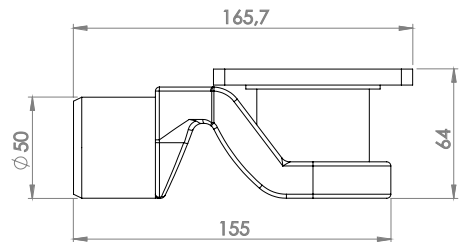
Yan Görünüm
