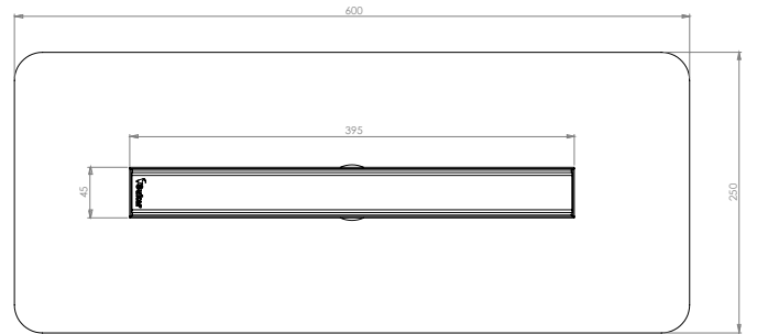
Üst Görünüm
