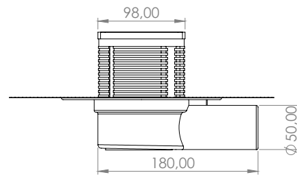
Yan Görünüm
