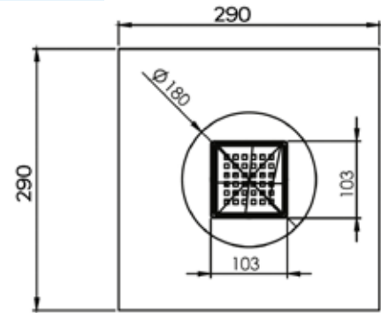
Üst Görünüm
